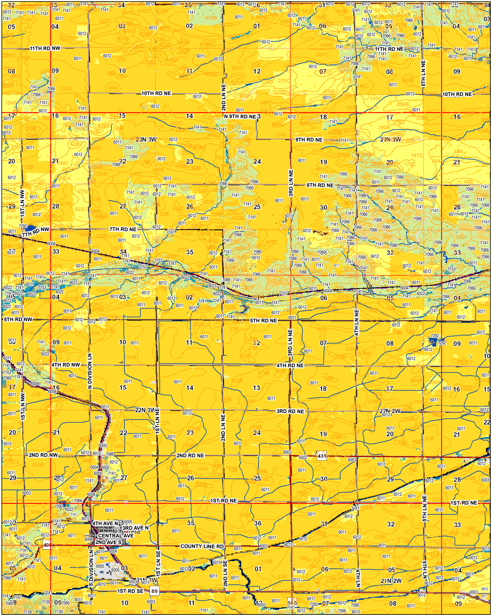
47111f8 - Cleiv
